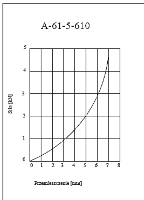
Charakterystyka statyczna
