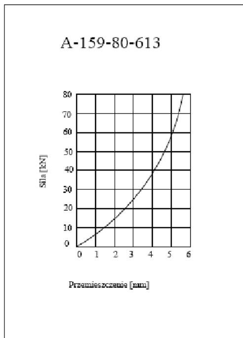
Charakterystyka statyczna
