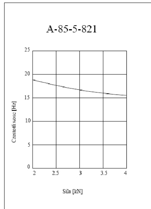
Charakterystyka dynamiczna
