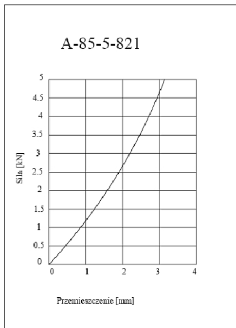
Charakterystyka statyczna
